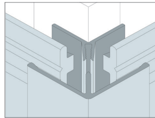
Eck-Profil (2-teilig)
