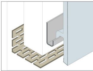
Starterleiste & Lüftungsprofil
