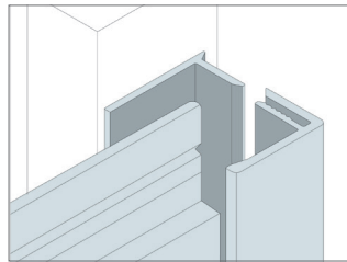
U-Profil (2-teilig)
